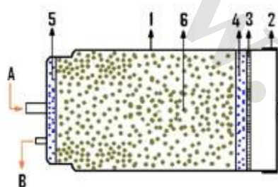
شکل 2- طرح کلی کنیستر و المان های اصلی
