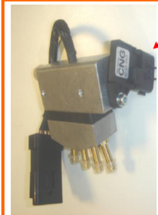
سنسور فشار- دمای گاز TMap Gas
