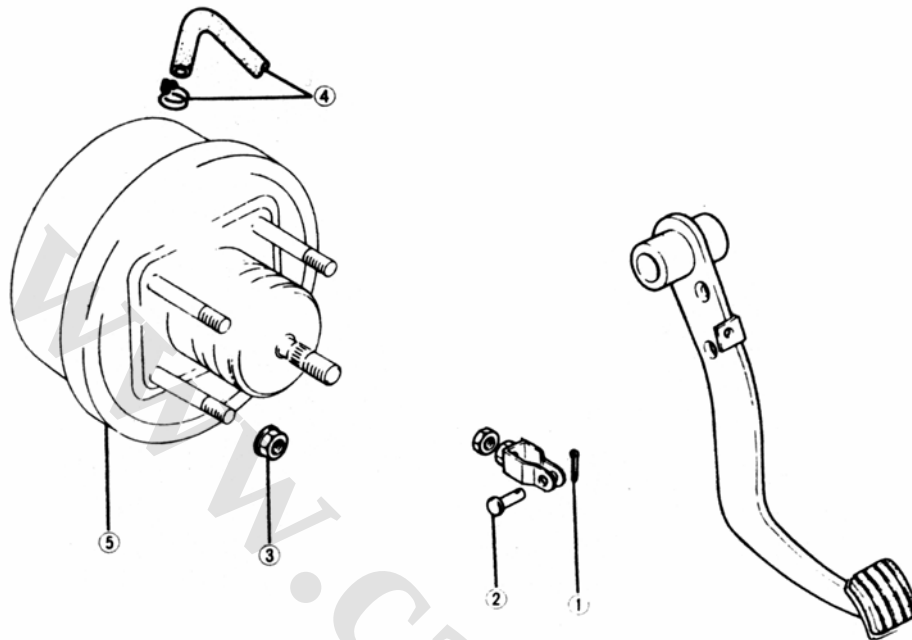
۵- بوستر ترمز
