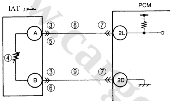
سنسور IAT
