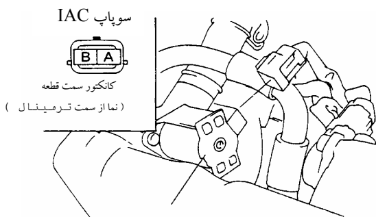
سوپاپ IAC
