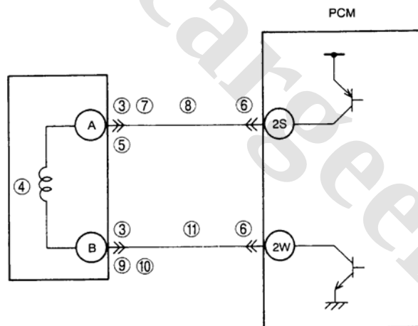
سوپاپ IAC
