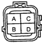
کانکتور سمت سیم کشی (نما از سمت ترمینال)
