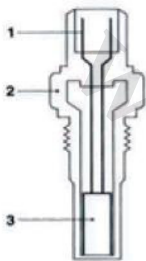
دیاگرام ساختار
