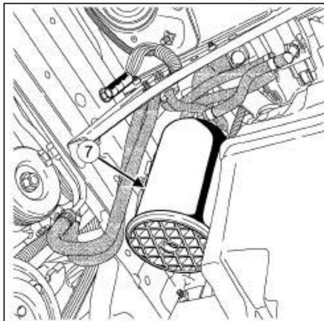
(7) جاذب بخارات بنزین
