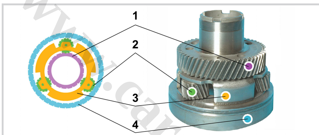
شکل ۱۹. مجموعه چرخ دنده سیاره‌ای ساده
