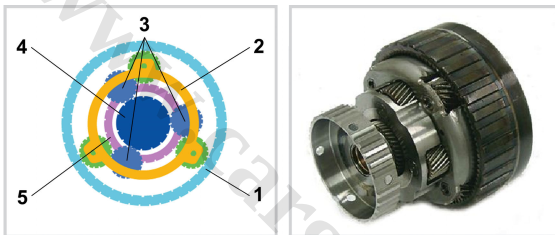
شکل ۲۰. مجموعه چرخ دنده سیاره‌ای مرکب.
