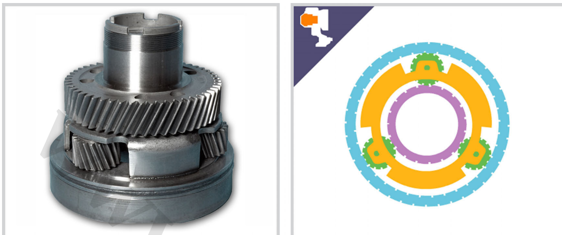
شکل ۱۰. چرخ‌دنده‌های سیاره‌ای.
