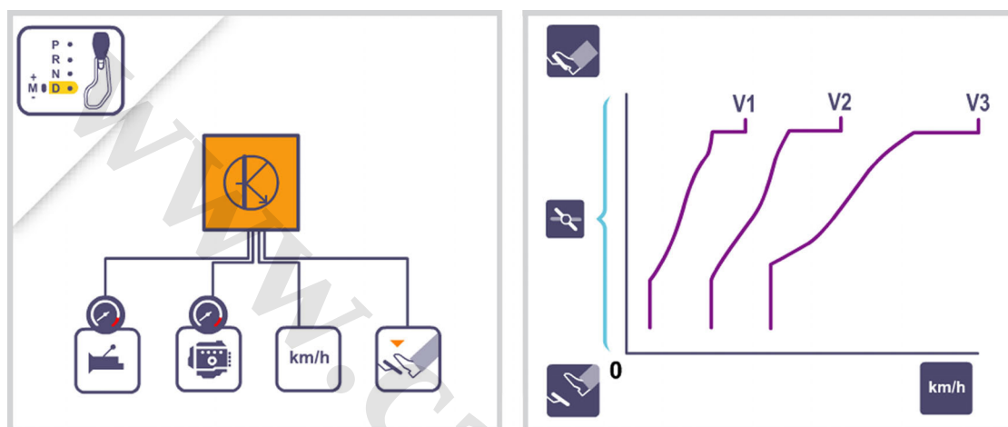
شکل ۴۰. برنامه ریزی واحد کنترل الکترونیکی گیربکس اتوماتیک.
