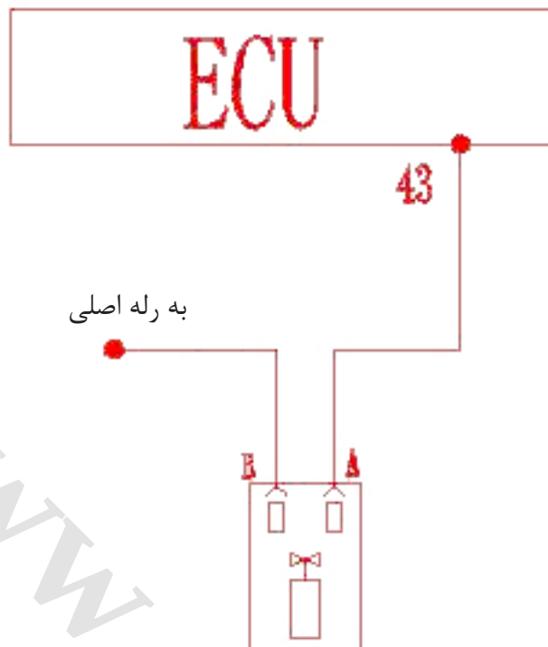
سوپاپ پالایش کربن گیر نمودار مدار سوپاپ پالایش کربن گیر
