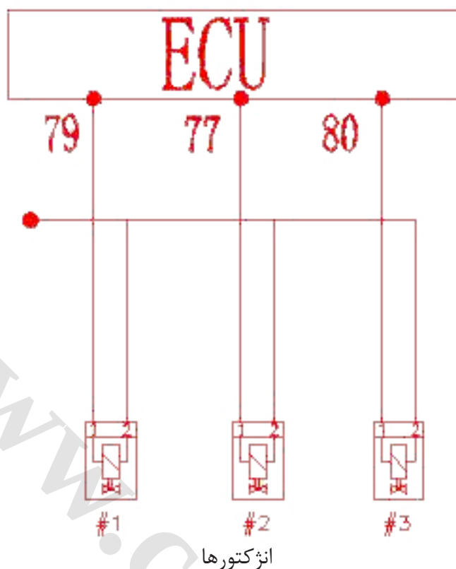
نمودار مدار انژکتور الکترومغناطیسی
